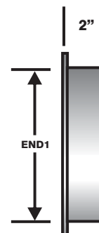
END CAP
