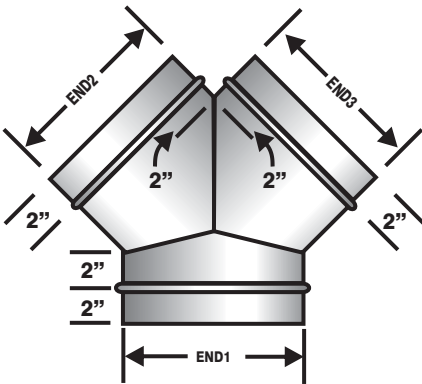
Y BRANCH
